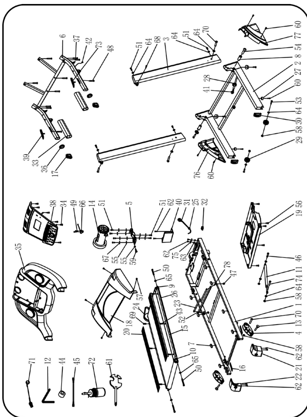
Схема тренажера в разобранном виде
